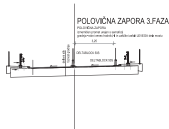
faza 3. gradnje prečni prerez B - B
