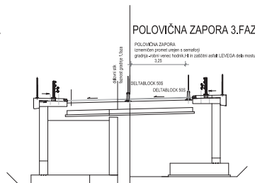
faza 3. gradnje prečni prerez A - A, C - C
