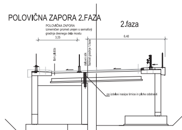
faza 2. gradnja desnega dela mostu prečni prerez A - A, C - C
